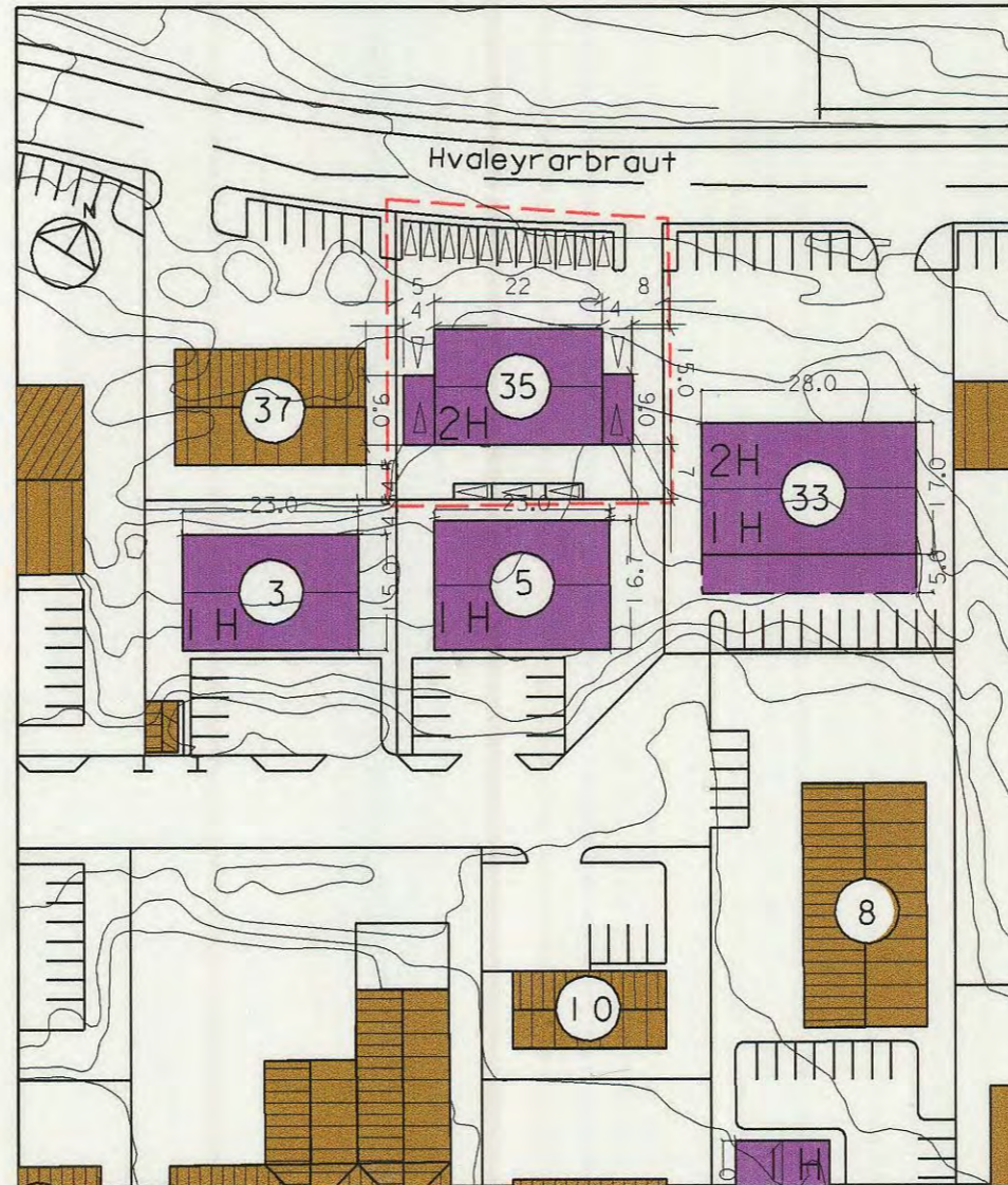
Deiliskipulag eftir breytingu. Mk 1:500
